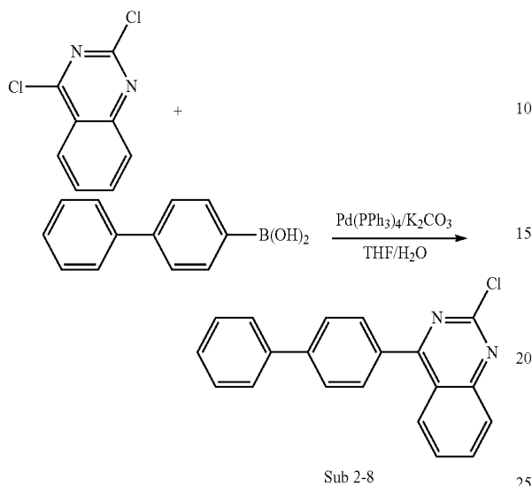
&lt;Reaction Scheme 12&gt;
